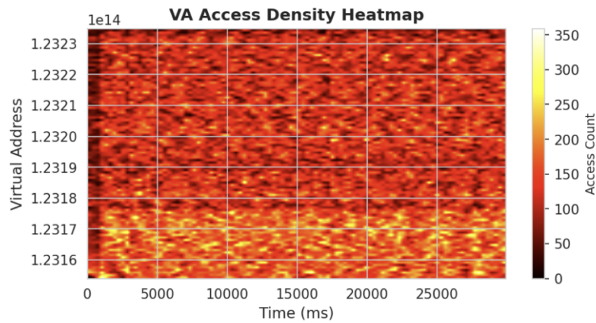
FAISS Query
