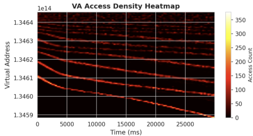
FAISS Build
