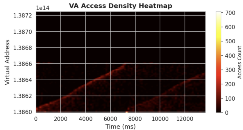
LLaMA Decode
