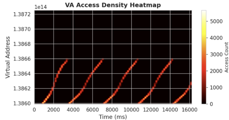
LLaMA Prefill
