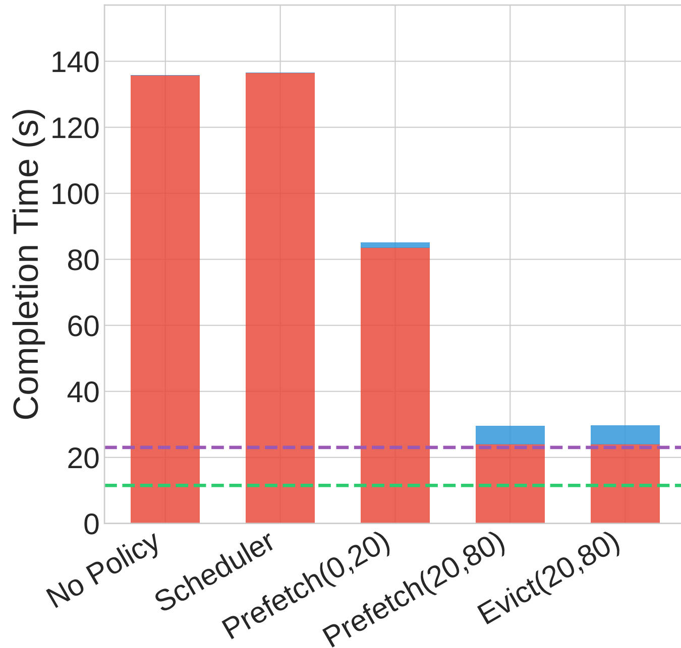
GEMM
