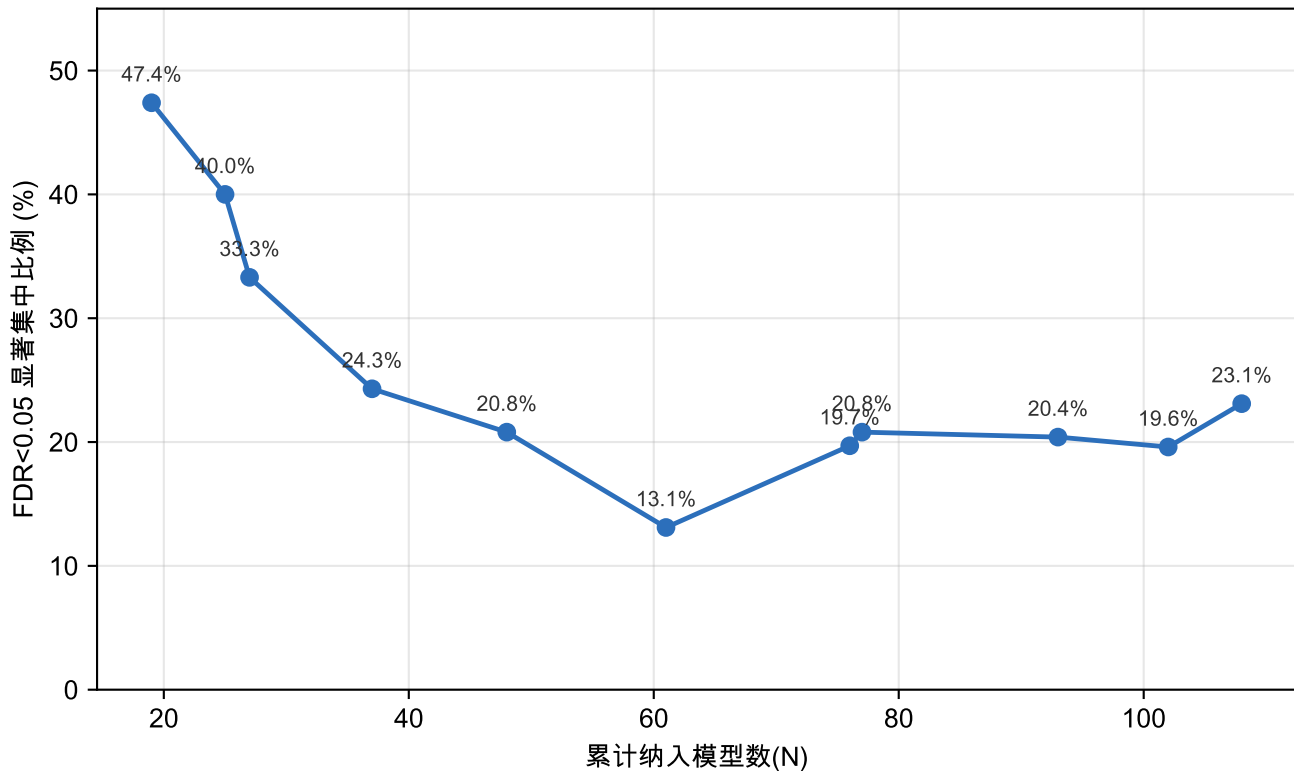
图2. 显著集中比例随样本规模变化的完整轨迹(11个checkpoint)
