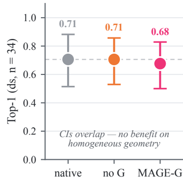
B. Reverse transfer ( \Delta = -0.029 , n.s.)
