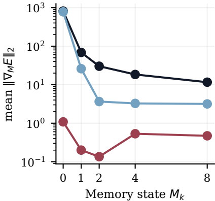
Local gradient norm
