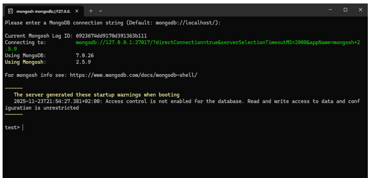
Рисунок 9.5 – Інтерфейс командного середовища MongoDB Shell
