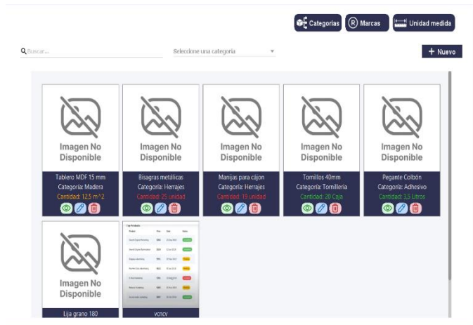
Vista Inventario
