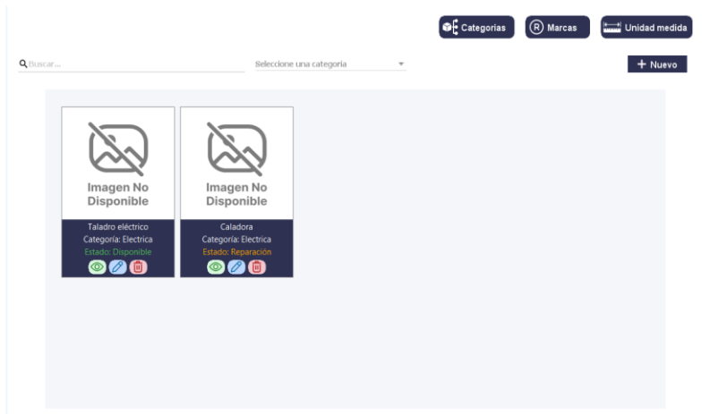
Vista herramientas
