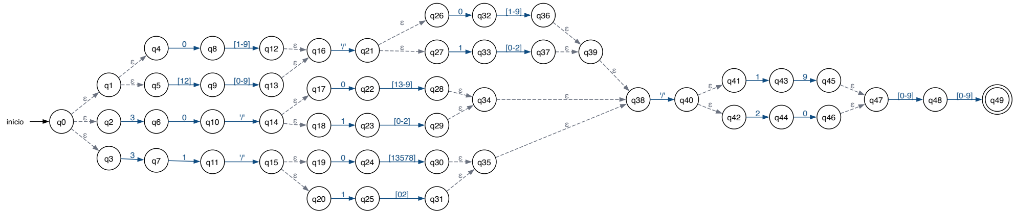
Figura 4 — AFNε de ER-04, gerado pela construção de Thompson a partir de ((0[1-9] \mid [12][0-9]) / (0[1-9] \mid 1[0-2]) \mid 30 / (0[13-9] \mid 1[0-2]) \mid 31 / (0[13578] \mid 1[02])) / (19 \mid 20)[0-9]\{2\} . Versão ampliada: docs/afn/er-04-data.svg.
