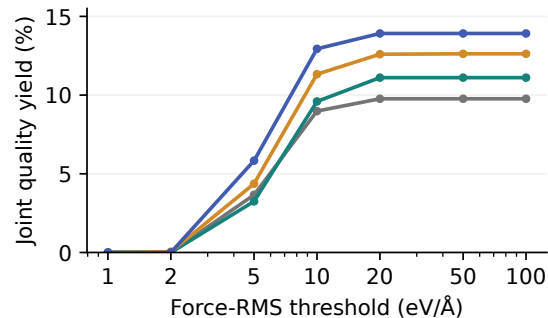
eSEN
