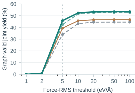
a eSEN
