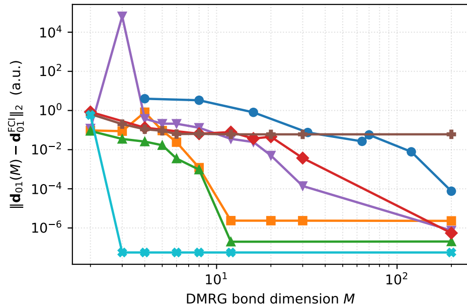
(b) Analytic NAC error (states 0,1)
