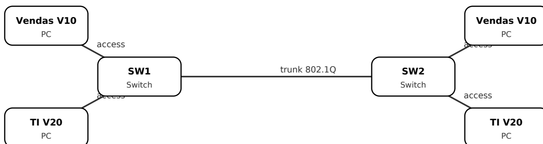
Figura: O trunk transporta várias VLANs no mesmo cabo, marcando cada trama com a etiqueta (tag) da VLAN.
