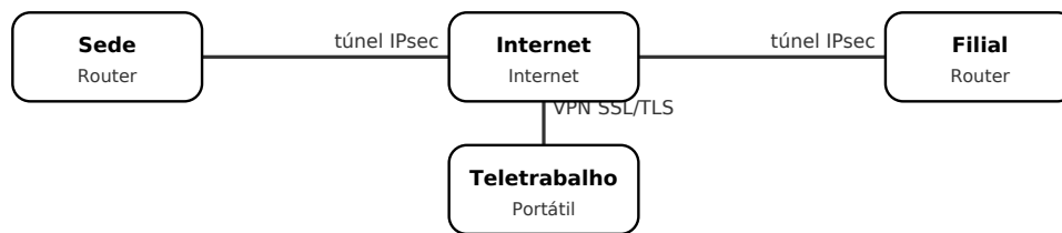
Figura: Site-to-site liga redes; acesso remoto liga um utilizador.
