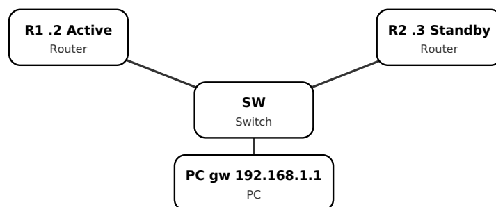
Figura: O PC usa o IP virtual 192.168.1.1.
