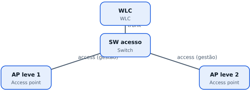
Figura: APs leves falam com a WLC por túneis CAPWAP (UDP 5246 controlo, 5247 dados).
