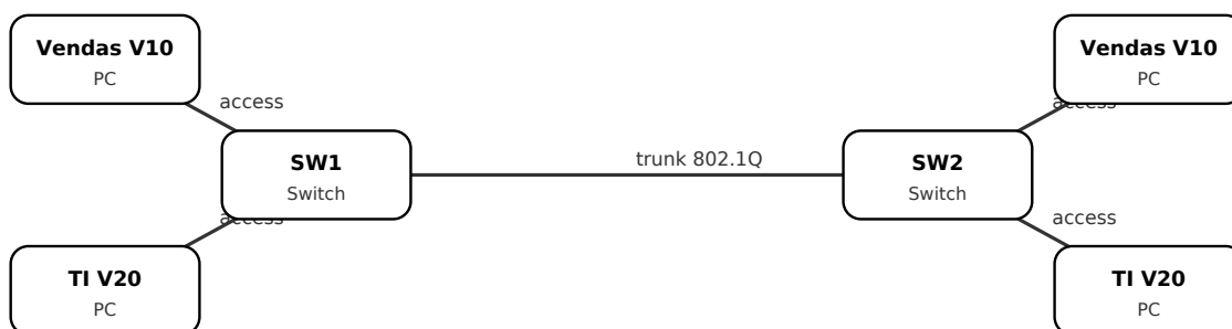
Figura: O trunk transporta várias VLANs no mesmo cabo, marcando cada trama com a etiqueta (tag) da VLAN.
