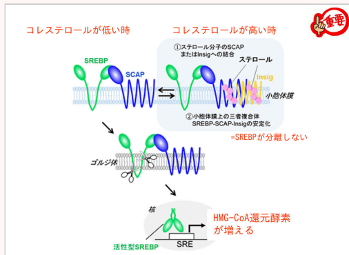
スライド6の図 (SREBPによる調節)
