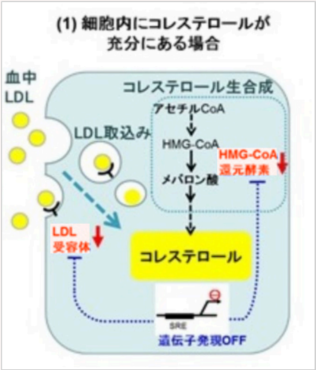
スライド14の図
