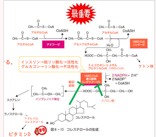
スライド6の図6-10(コレステロールの生成)
