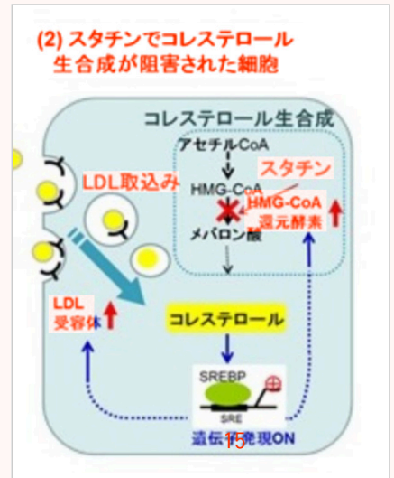
スライド15の図(スタチンでコレステロール生合成が阻害された細胞)
