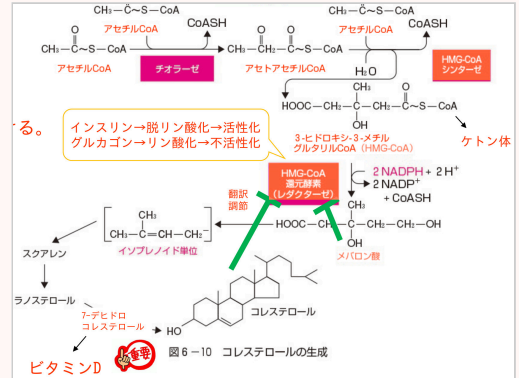
スライド6の図6-10(コレステロールの生成)
