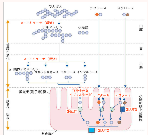
スライド18の図(薄い青の六角形=グルコース、橙の六角形=ガラクトース、茶色の五角形=フルクトース)
