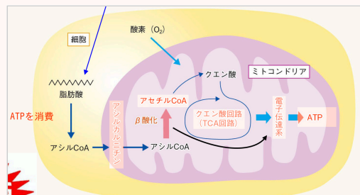
スライド11の概略図(脂質の細胞内代謝)
