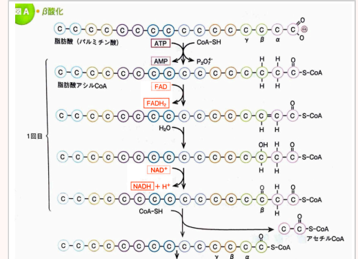
スライド13の図(パルミチン酸の1回目の \beta 酸化)
