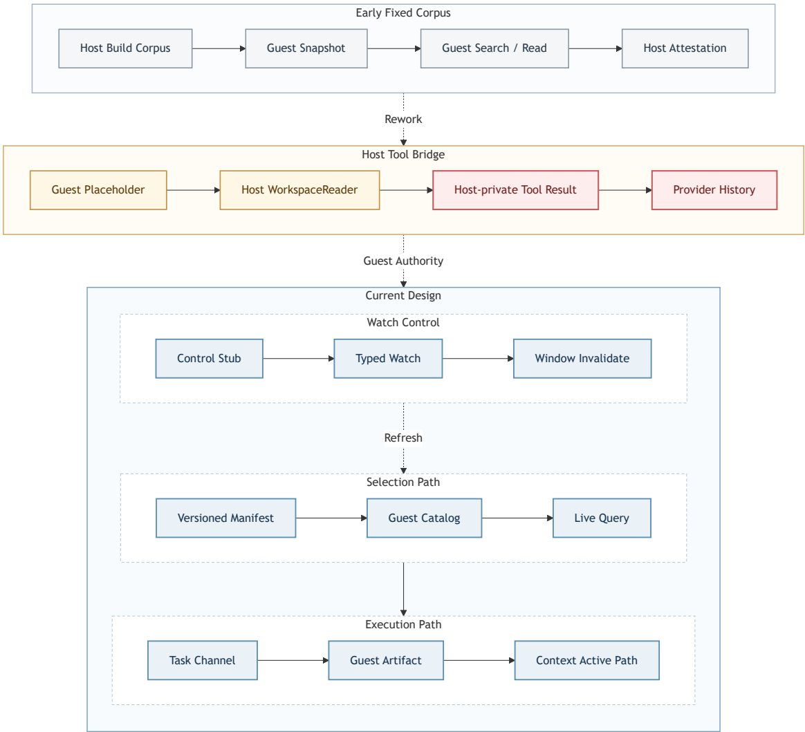
图 3.13: Nexus 从 Host 语义分散收敛为 Guest 权威、Host 代理
