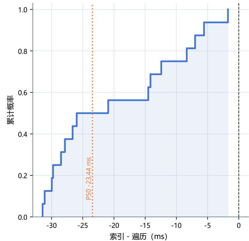
配对差值 ECDF
