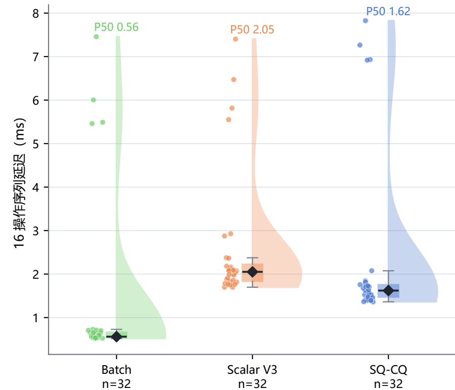
延迟雨云图
