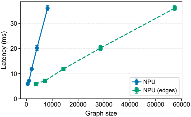
APPNP_fp32
