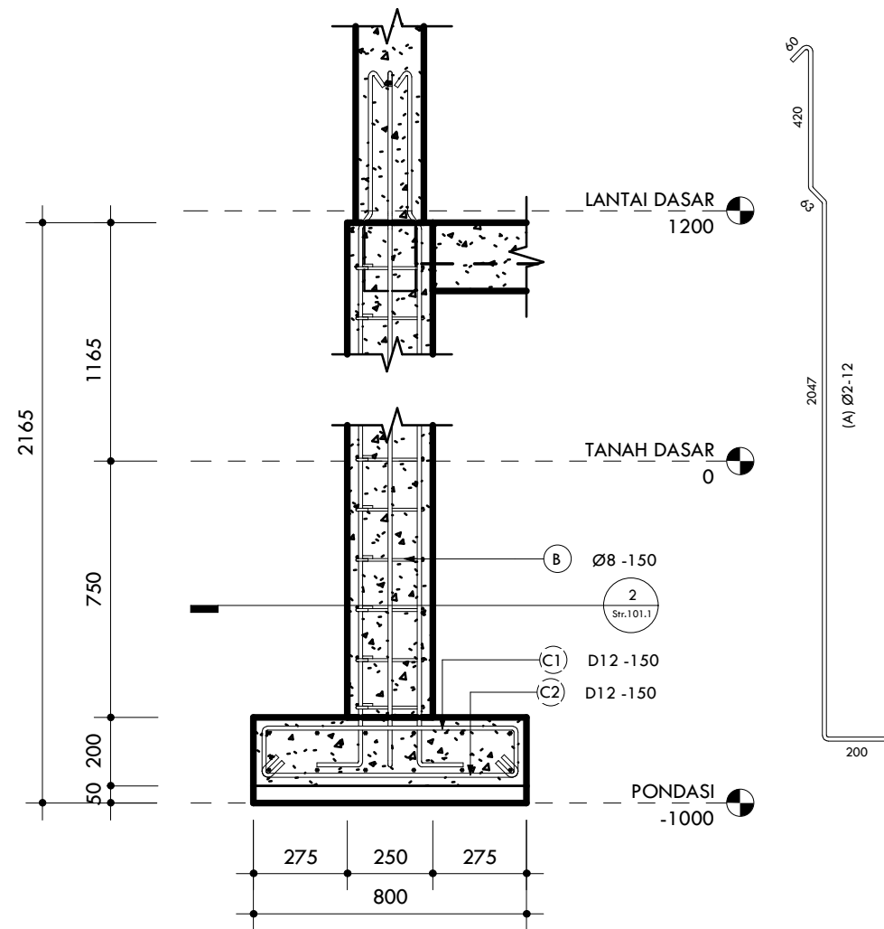
1 DETAIL POTONGAN PONDASI P1 1 : 20
