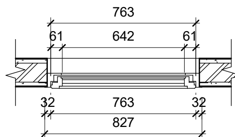
8 DETAIL J4 - ATAS 1 : 20
