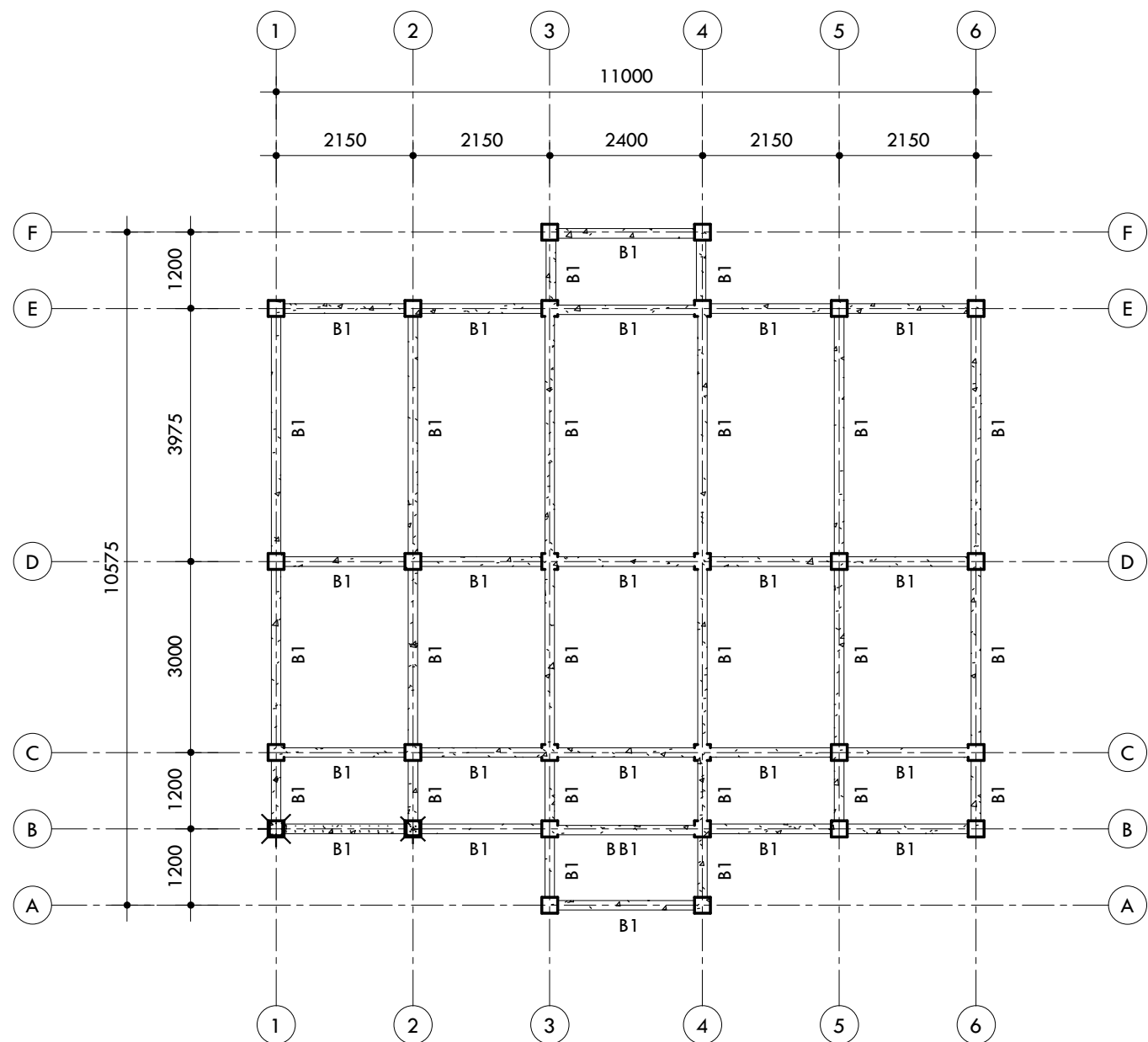
1 DENAH BALOK ELV +1.200 1 : 100
