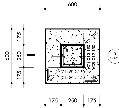
4 DETAIL TAPAK PONDASI P2 1 : 20
