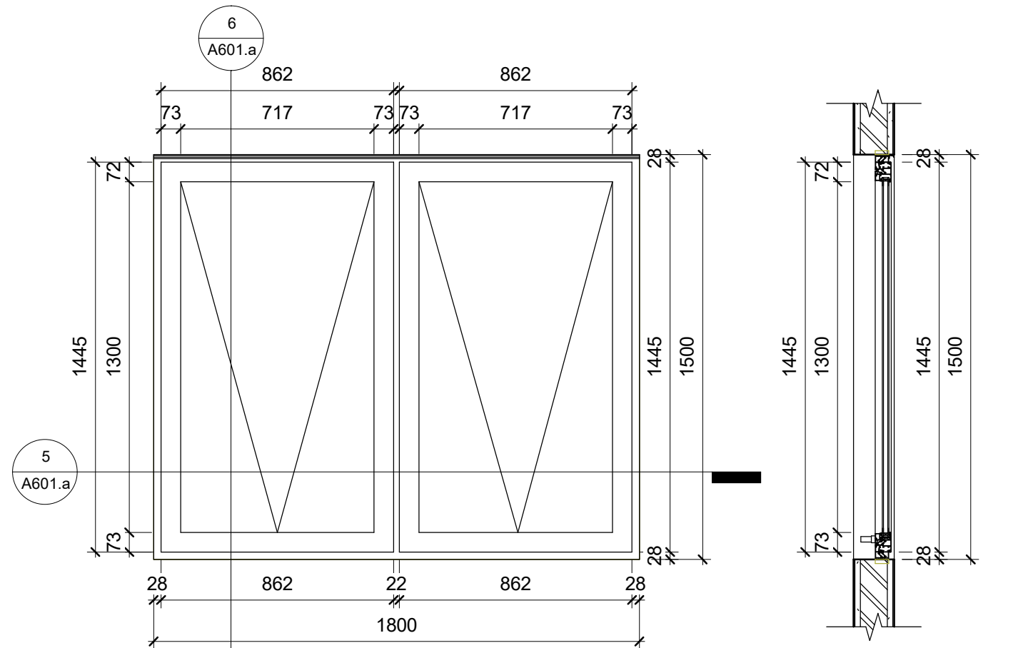
4 DETAIL J1 - DEPAN 1 : 20
