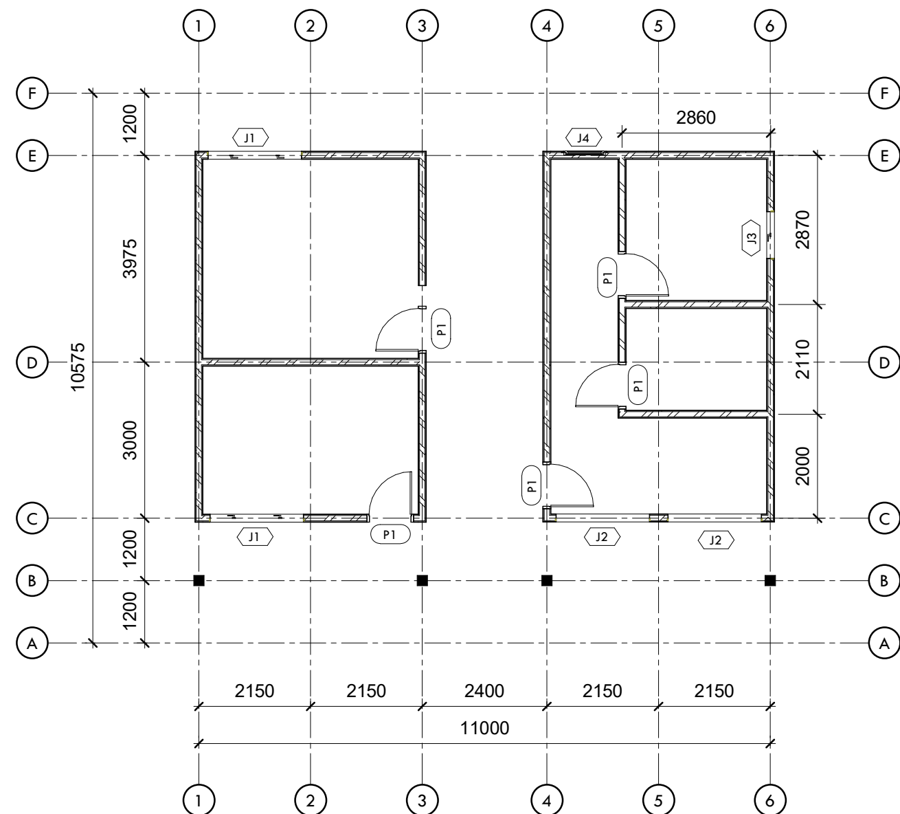
1 DENAH RENCANA PINTU DAN JENDELA 1 : 100
