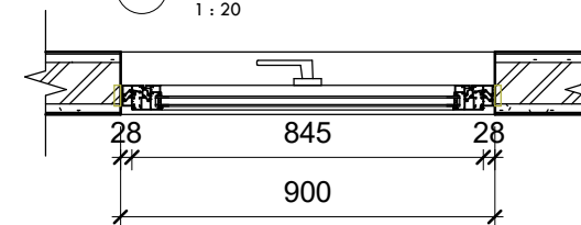
5 DETAIL J3 - ATAS 1 : 20
