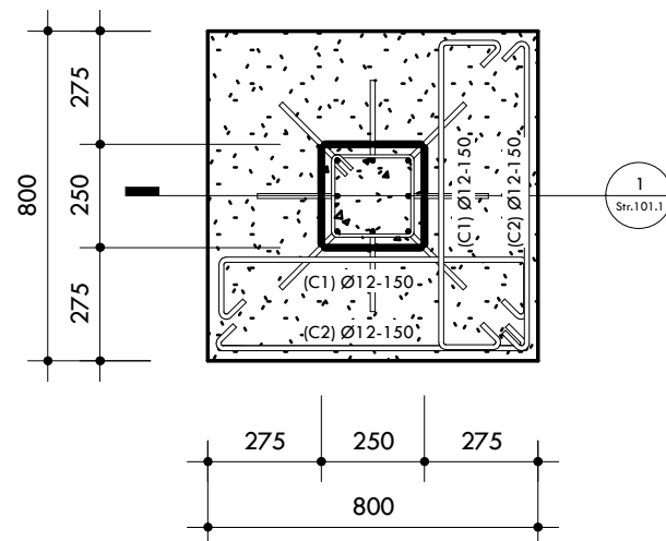
2 DETAIL TAPAK PONDASI P1 1 : 20
