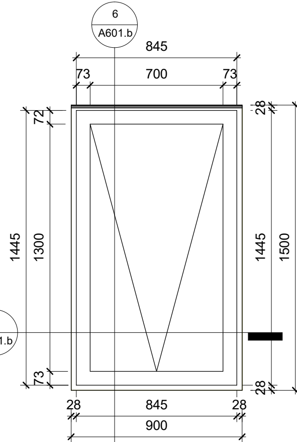
4 DETAIL J3 - DEPAN 1 : 20
