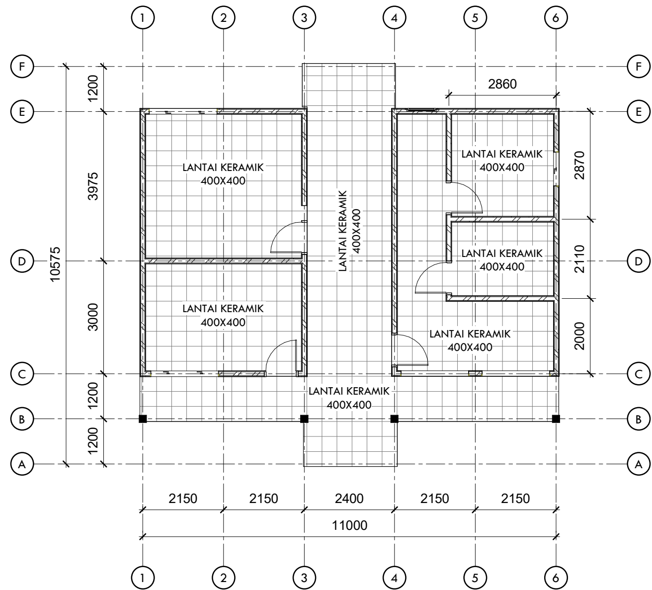
1 DENAH RENCANA LANTAI KERAMIK 1 : 100
