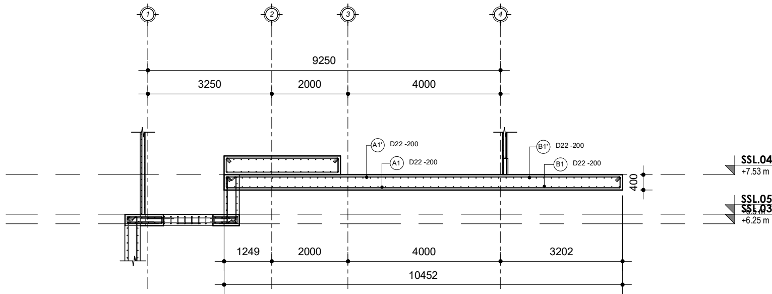
1 Potongan A - Slab Lantai 1 : 100
