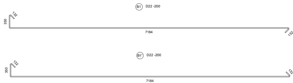
1 Potongan B - Wall Structure 1 : 50
