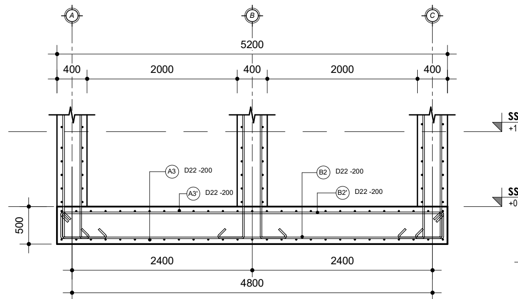
2 Potongan C - Floor Slab 1 : 50
