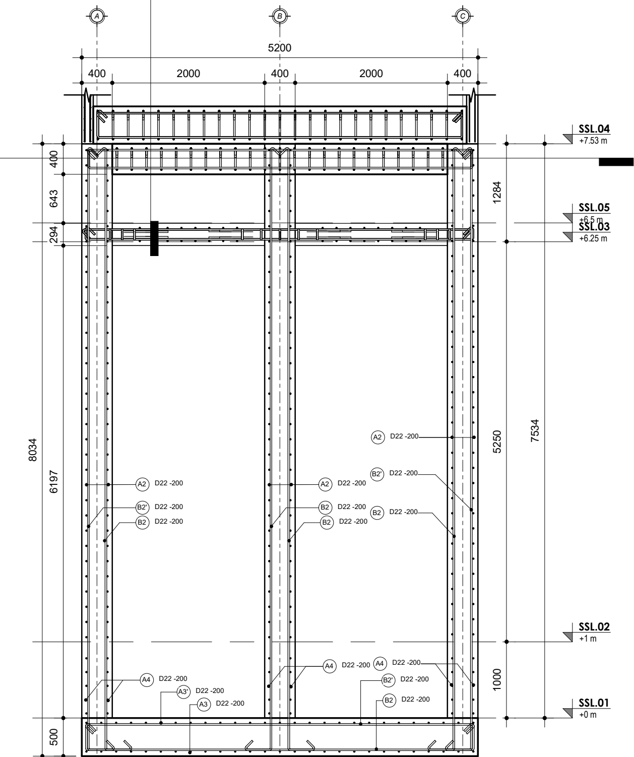
2 Potongan C - Wall Structure 1 : 50
