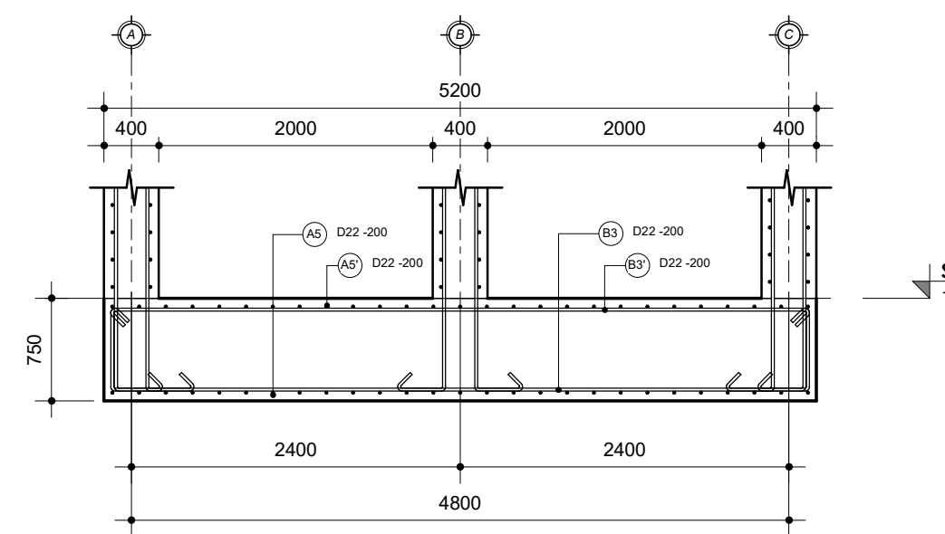
3 Potongan D - Floor Slab 1 : 50
