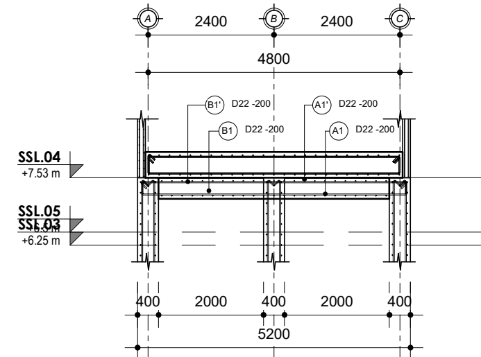
2 Potongan C - Slab Lantai 1 : 100
