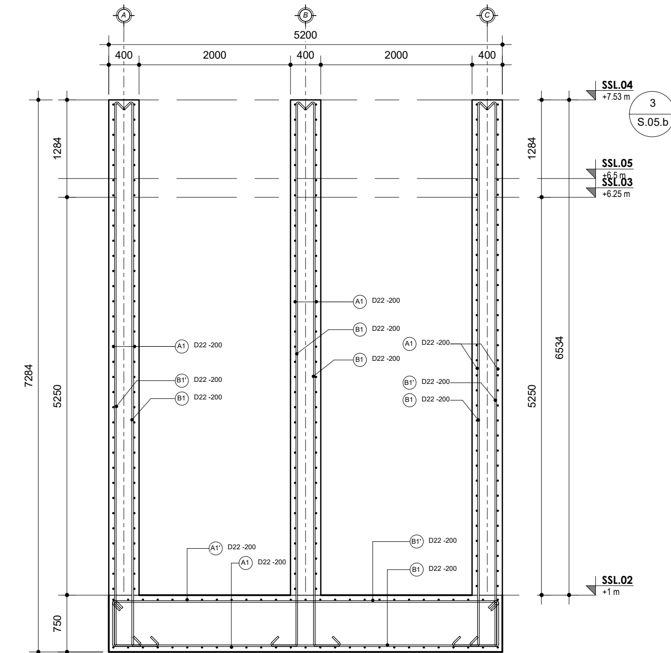
1 Potongan B - Wall Structure 1 : 50
