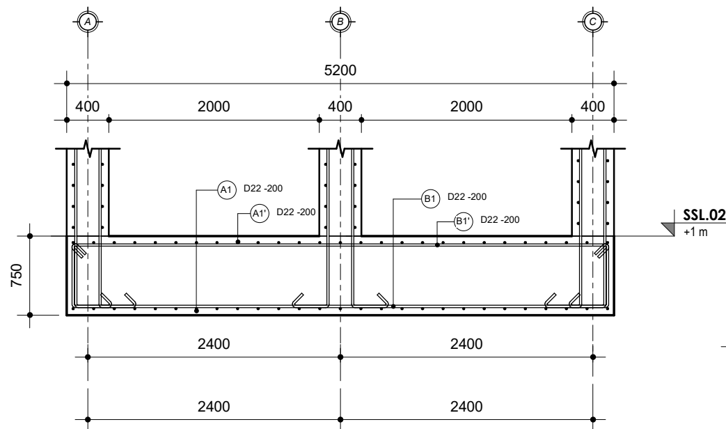
1 Potongan B - Floor Slab 1 : 50
