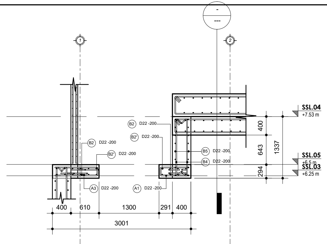
2 Potongan A - Slab Pompa 1 : 50
