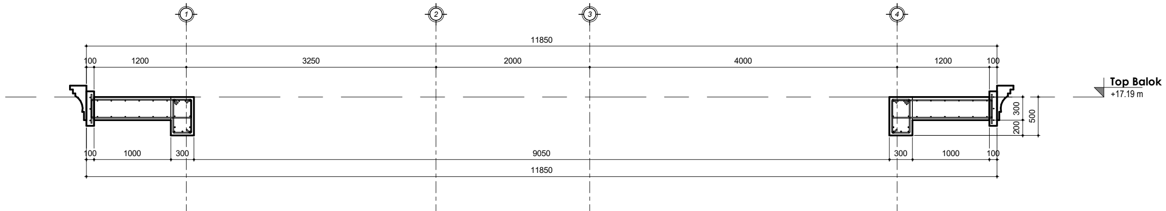
2 Detail Memanjang 2 1 : 50
