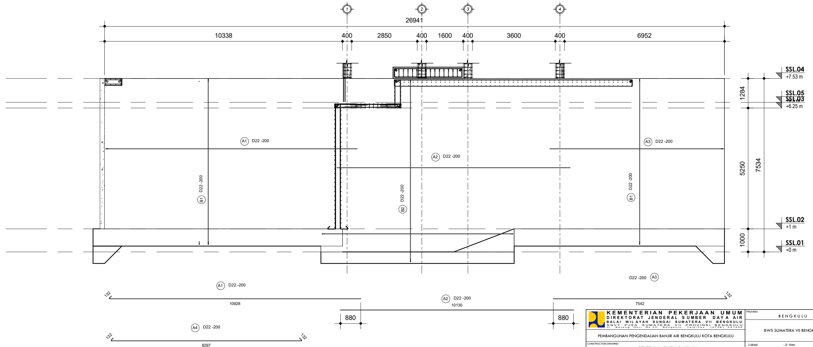
2 Potongan A - Wall Structure 1 : 100
