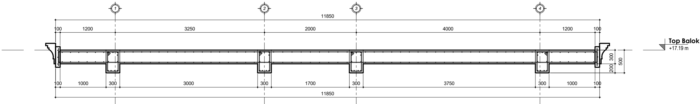
1 Detail Memanjang 1 1 : 50
