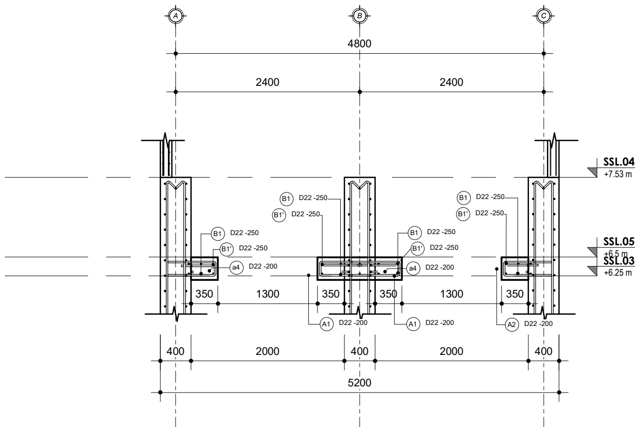
1 Potongan C - Slab pompa 1 : 50
