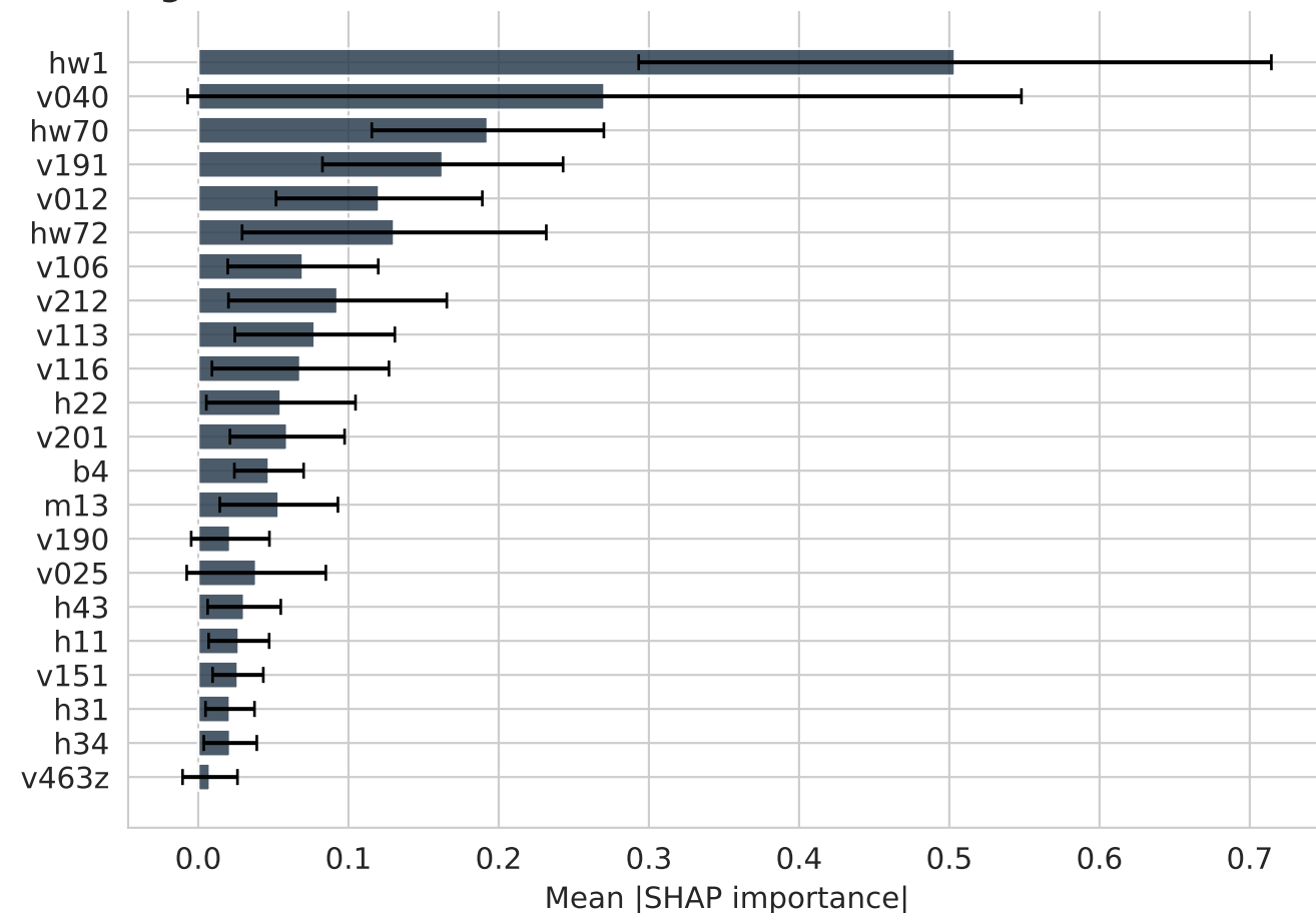
TabPFN
