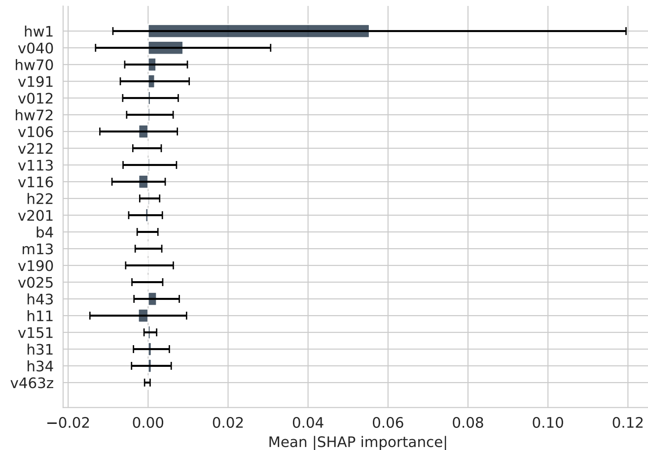
TabPFN
