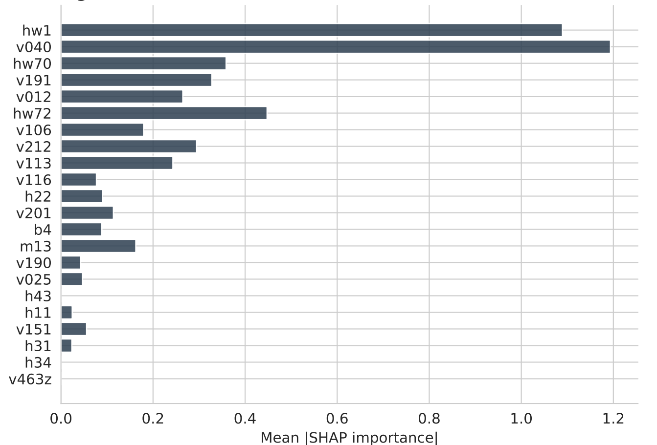
TabPFN
