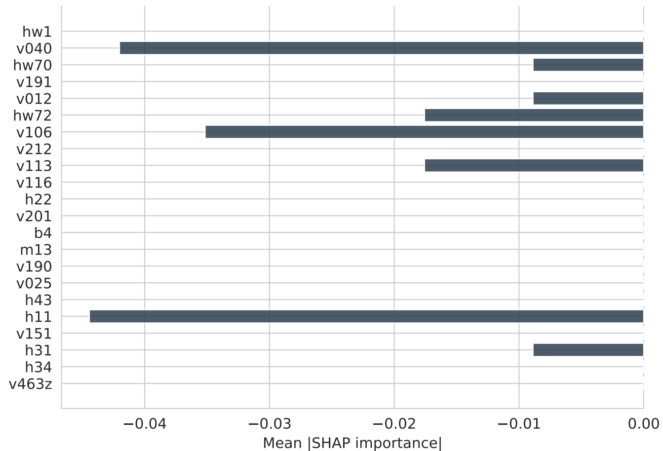
TabPFN
