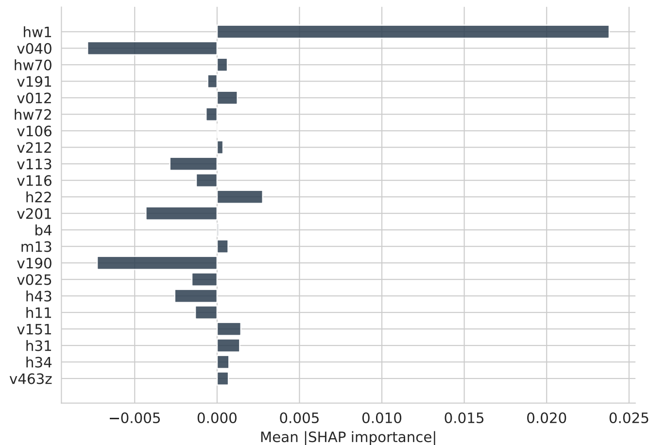
TabPFN
