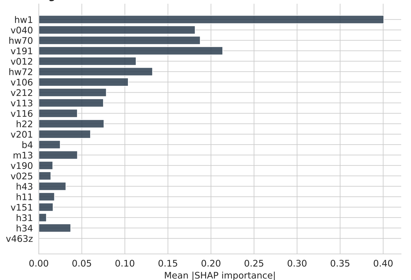
TabPFN
