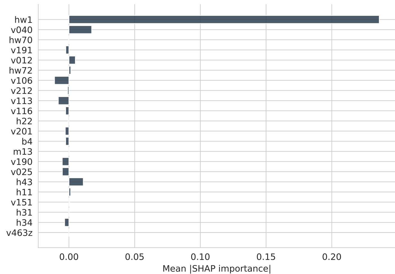
TabPFN
