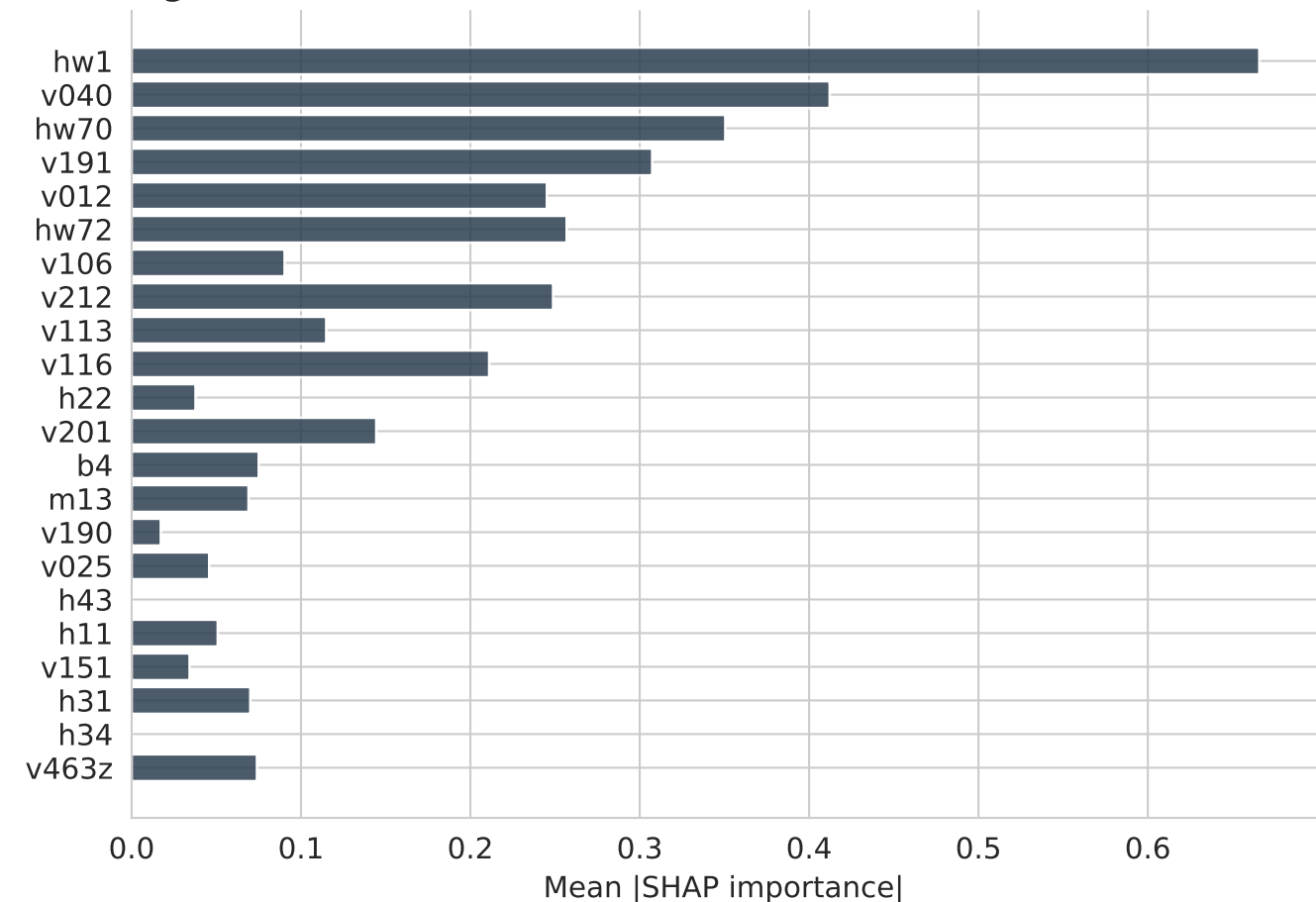
TabPFN
