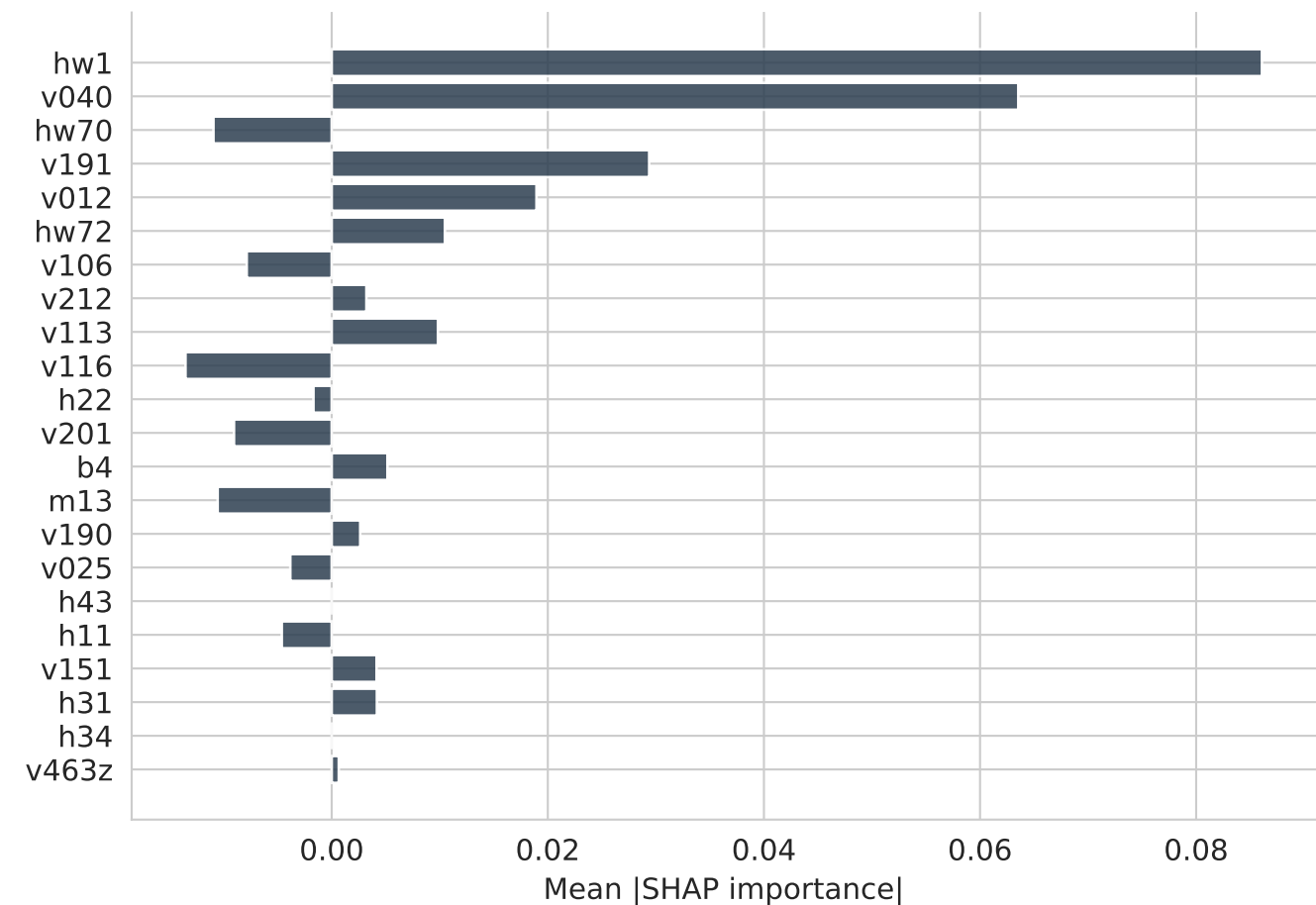
TabPFN
