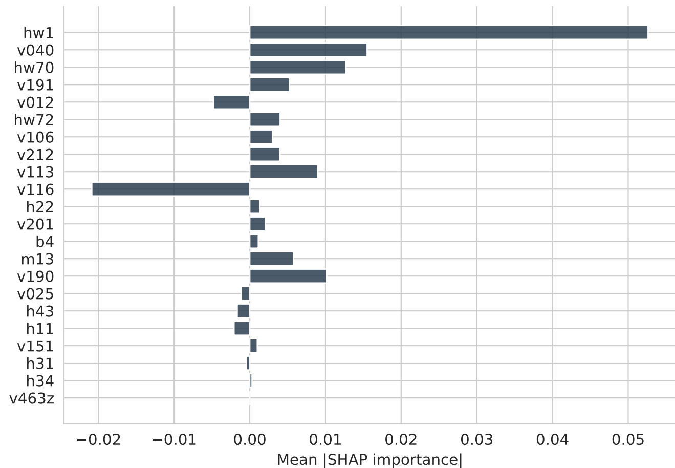
TabPFN
