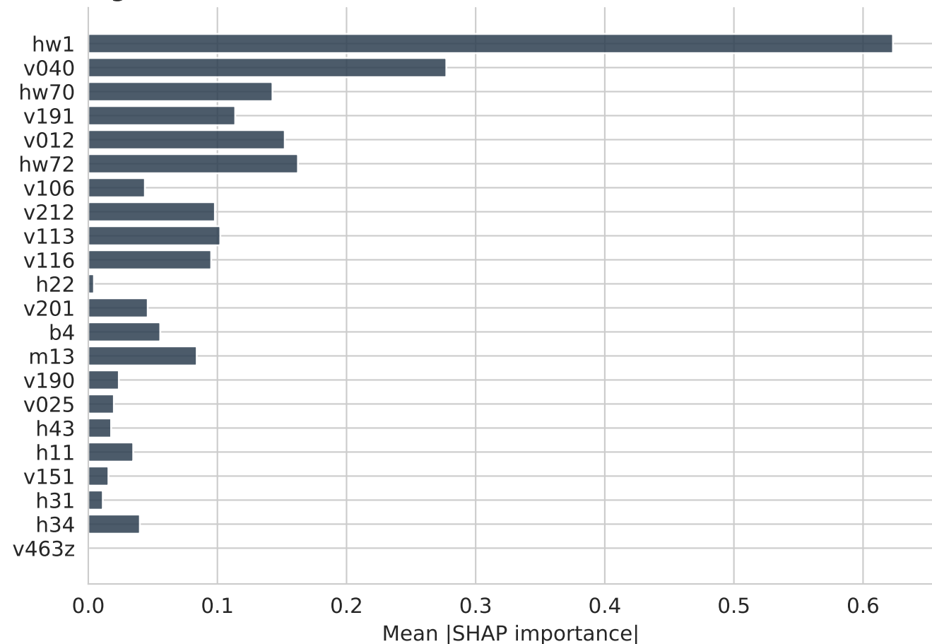
TabPFN
