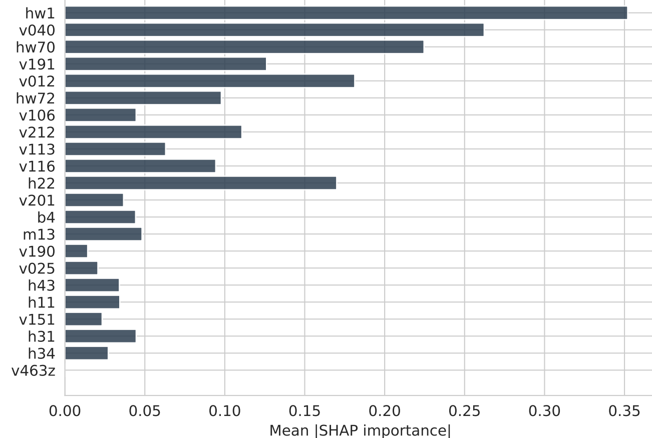
TabPFN
