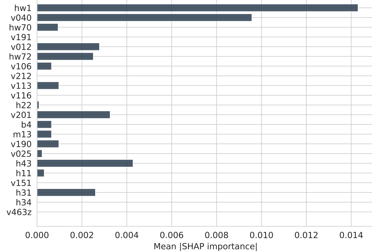
TabPFN
