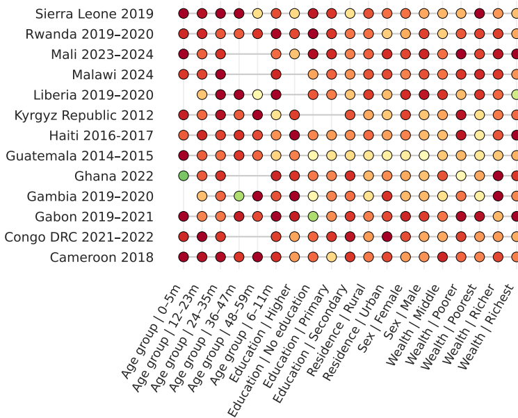
TabPFN
