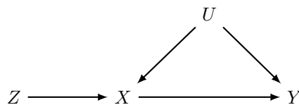
図 16 操作変数法
