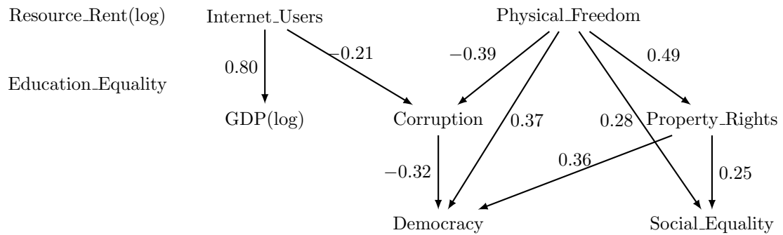
図 19 LiNGAM による政治経済指標の因果探索結果
