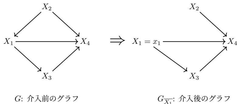
図 13 介入によるグラフの変化
