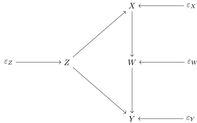
図 17 構造的因果モデル
