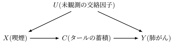
図 15 喫煙と肺がんの因果関係
