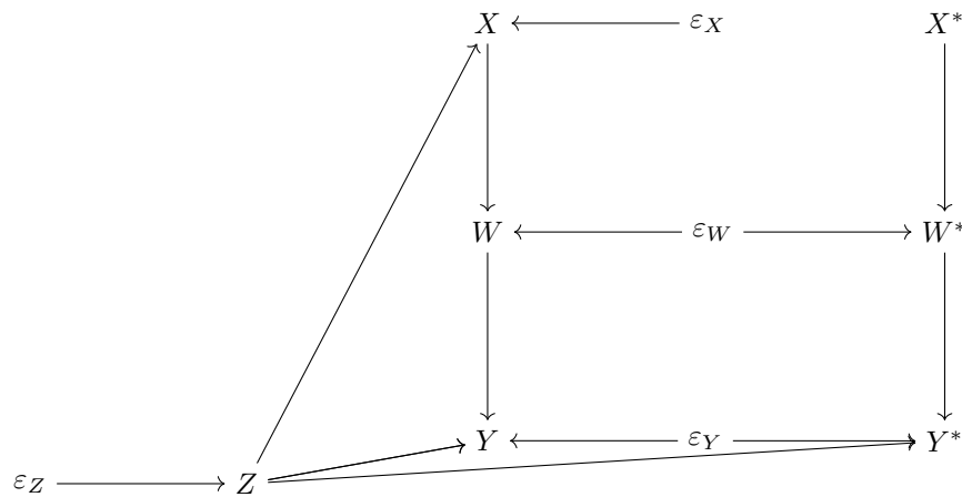
図 18 ツインネットワーク
