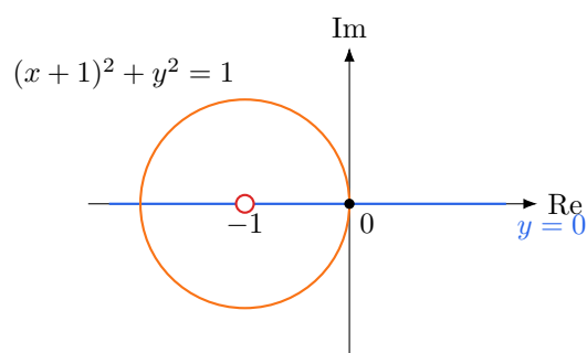
図 23: 軌跡は実軸と円 (x + 1)^2 + y^2 = 1 であり、 z = -1 は除く
