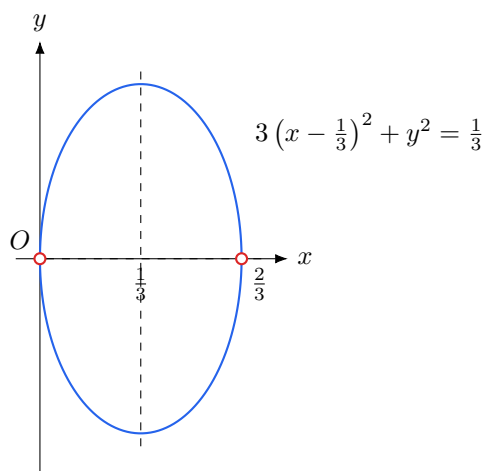
図 21: P の軌跡は楕円上の点であり, m \neq 0 のため x 軸上の 2 点は除く
