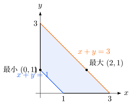
図 19: 条件 x \geq 0, y \geq 0, 1 \leq x + y \leq 3 が表す領域
