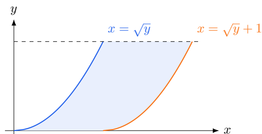
図 18: 0 \leq y \leq 1 の各高さで x が長さ 1 の区間を動く
