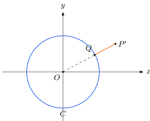
図 13: 点 P を平面 z = 0 に射影し、平面内で円との最短距離を調べる
