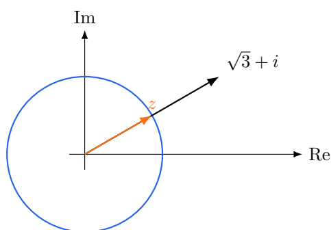
図 20: 同じ向きに足すと絶対値が最大になる
