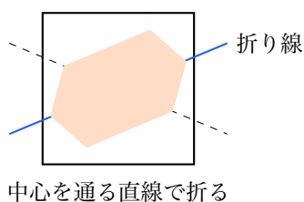
図 16: 折り線に沿った座標で, 反射後も正方形内に残る部分を調べる
