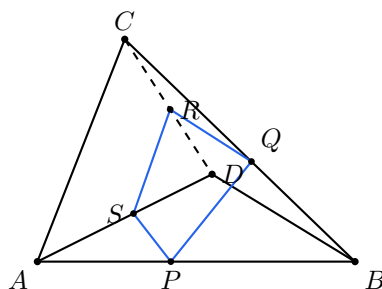
図 7: 辺上の4点 P, Q, R, S が同一平面上にある条件を調べる
