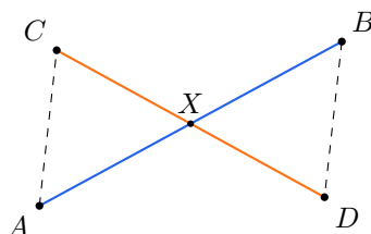
図 17: 交わる 2 線分は、組を替えると総延長を短くできる
