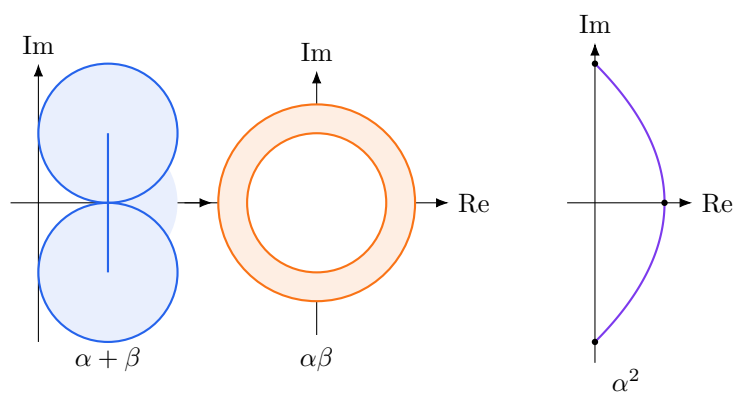
図 24: \alpha + \beta , \alpha\beta , \alpha^2 が描く範囲
