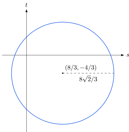
図 15: xy 平面上に現れる点 Q(s, t, 0) の軌跡
