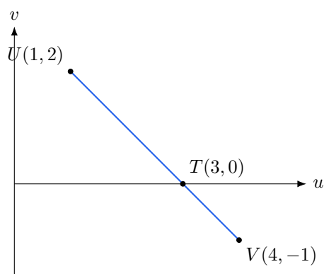
図 12: 空間内の 2 つの距離を補助平面上の折れ線 UT + TV に読み替える
