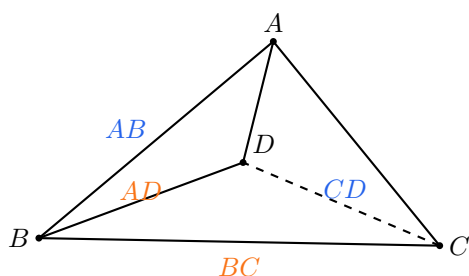
図 14: 等面四面体では向かい合う辺の長さが等しい
