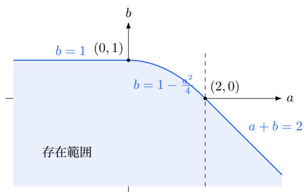
図 22: 円の中心 (a, b) の存在範囲は太線の下側である
