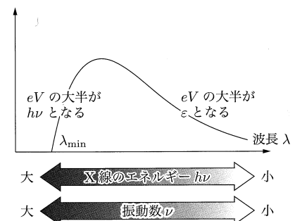
X線強度（光子数）
