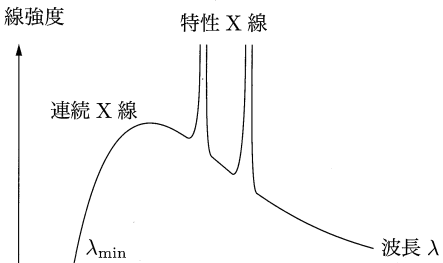
X線強度
