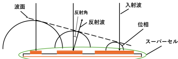
図 2 メタサーフェス反射板のスーパーセル Fig. 2. Supercell of the metasurface reflector.
