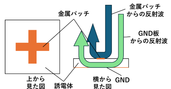
図 1 反射素子
