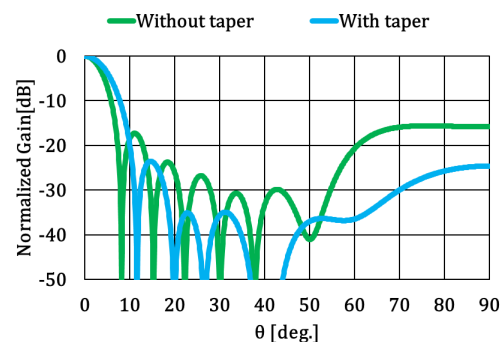
図1 -40dB テーパーとテーパーなしの特性比較 ( \varphi )
