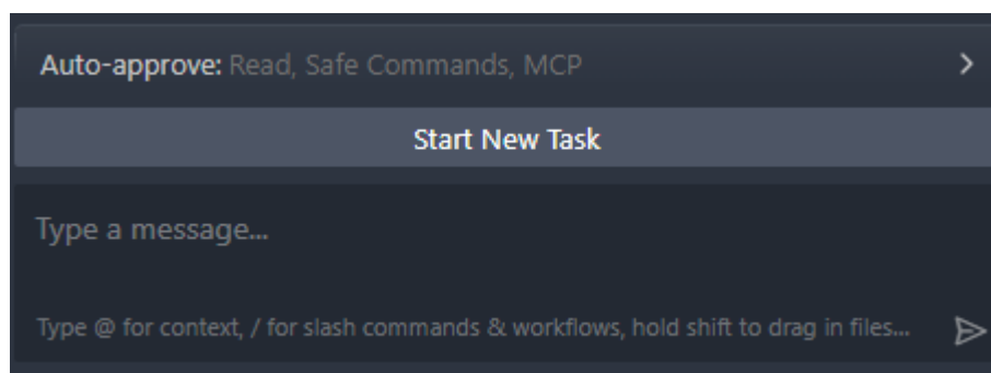
Рисунок 58 – Нижняя Cline
