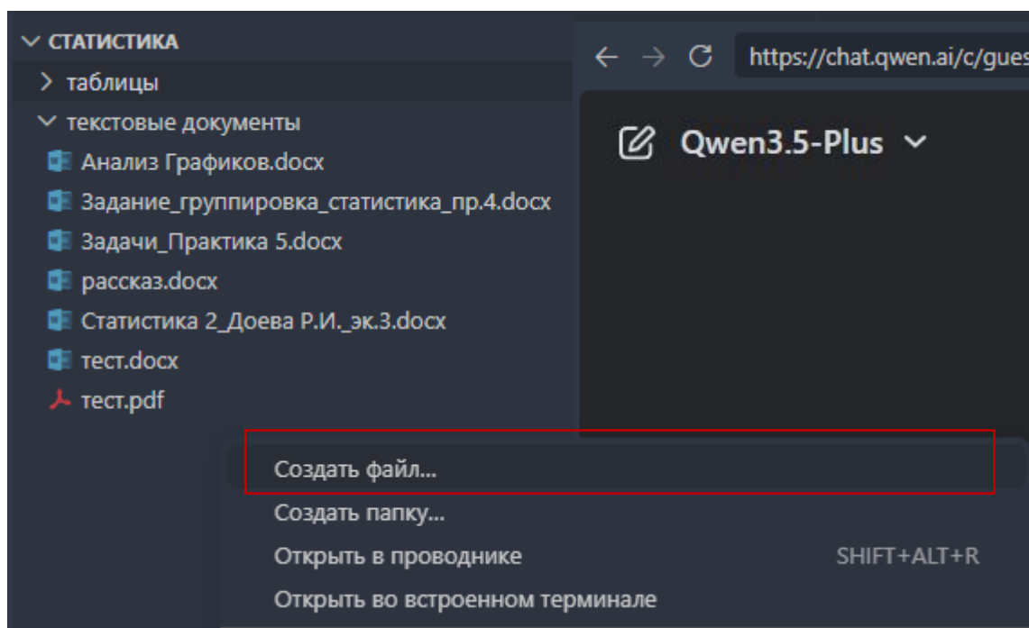
Рисунок 60 – Создание файла
