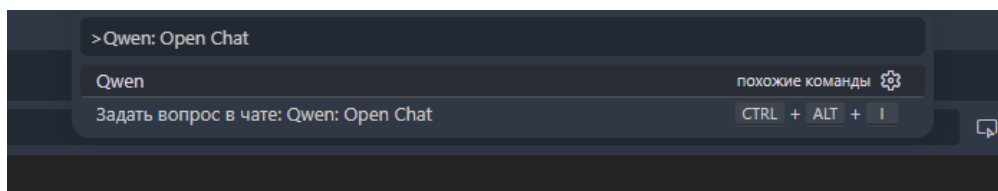
Рисунок 76 – Командная строка
