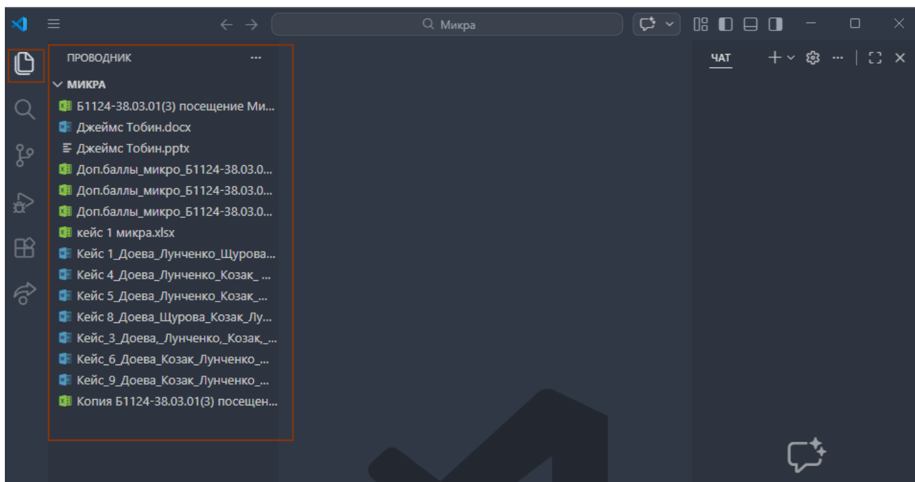
Рисунок 35 – Папка проекта
