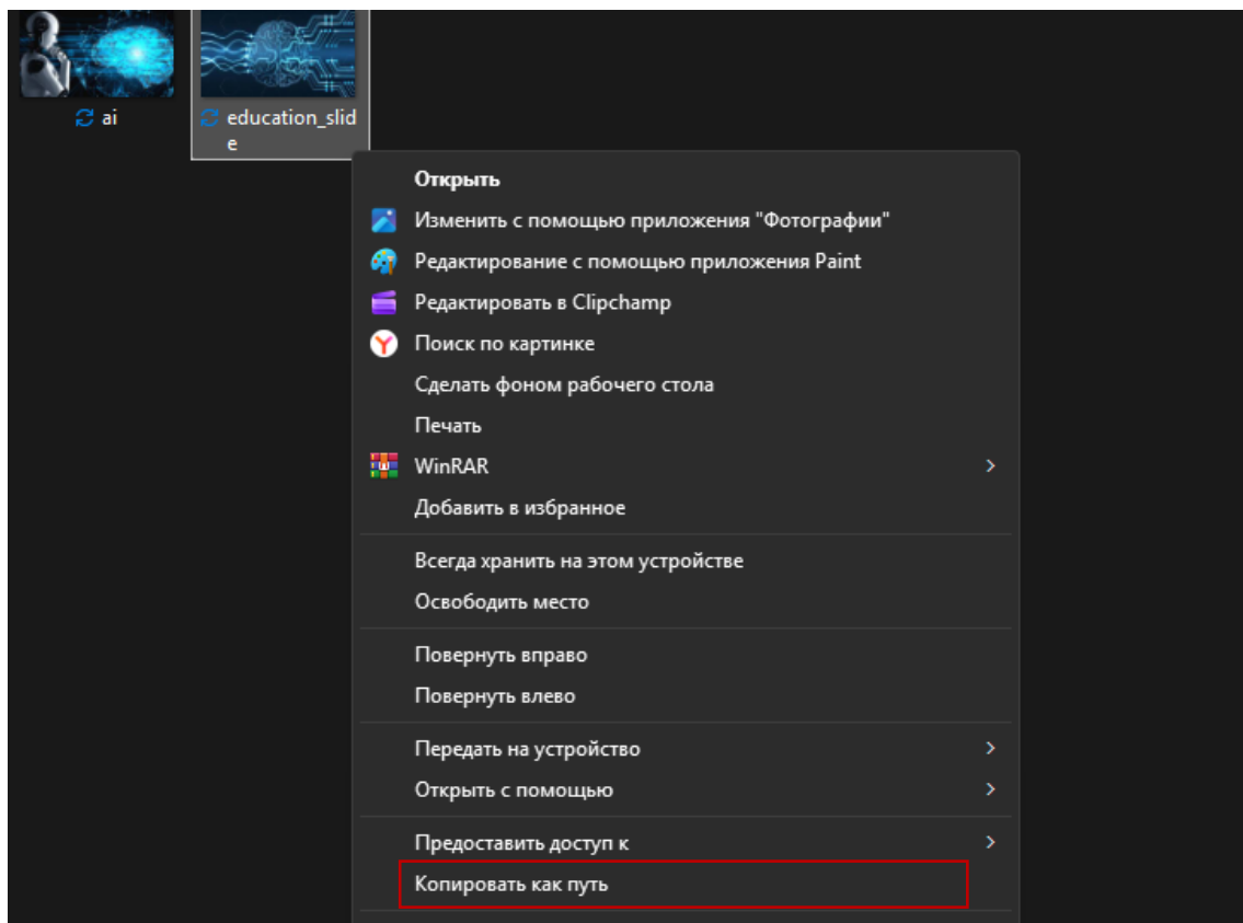
Рисунок 69 – Путь файла
