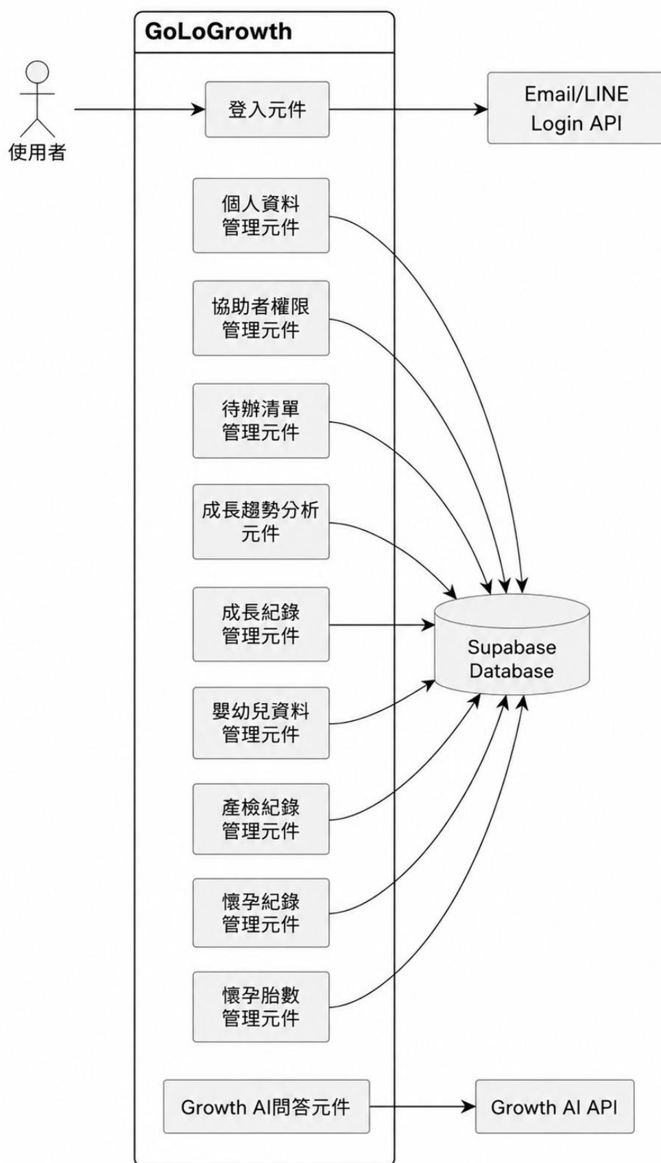
圖 7-3-1 元件圖
