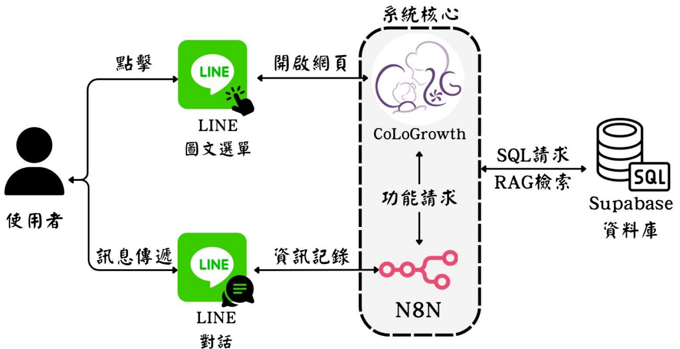
圖 3-1-1 系統架構圖
