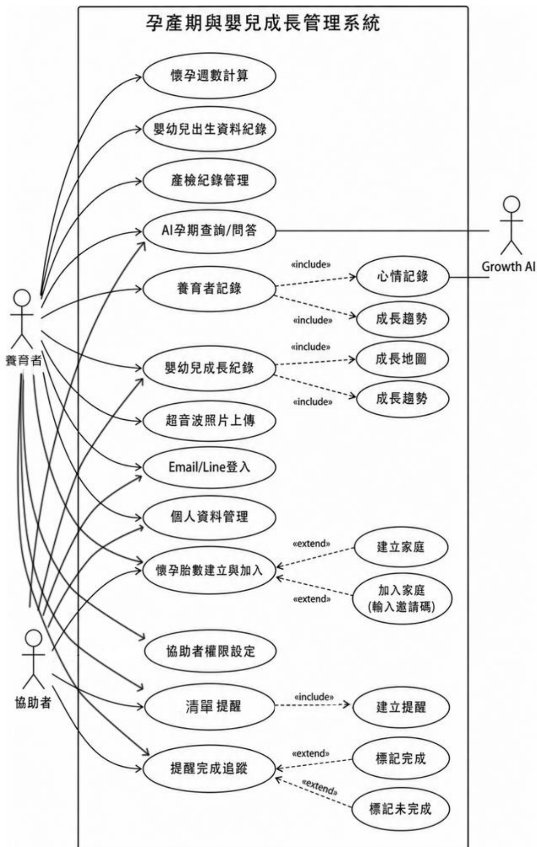
圖 5-2-1 使用個案圖
