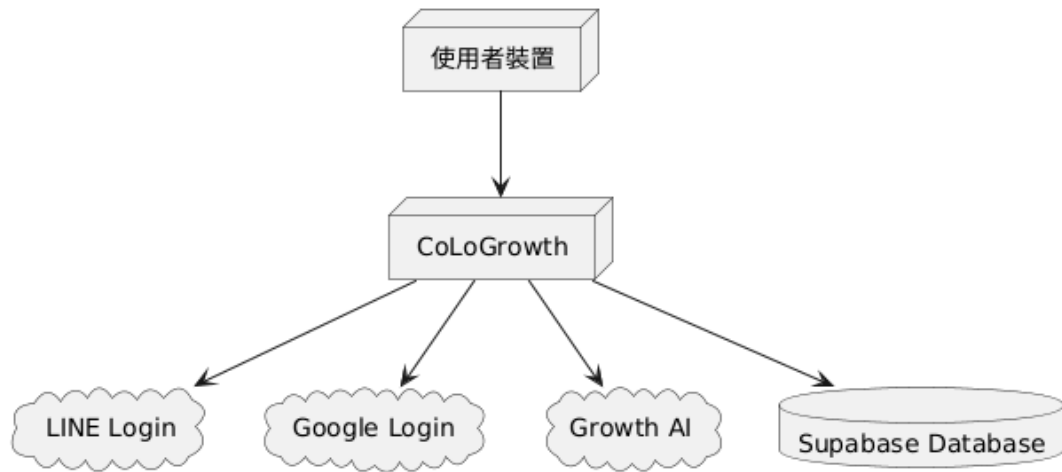
圖 7-1-1 佈署圖
