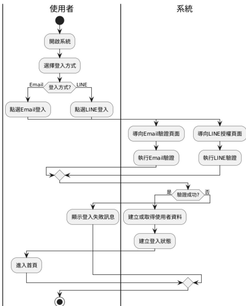
圖 5-3-1 註冊與登入
