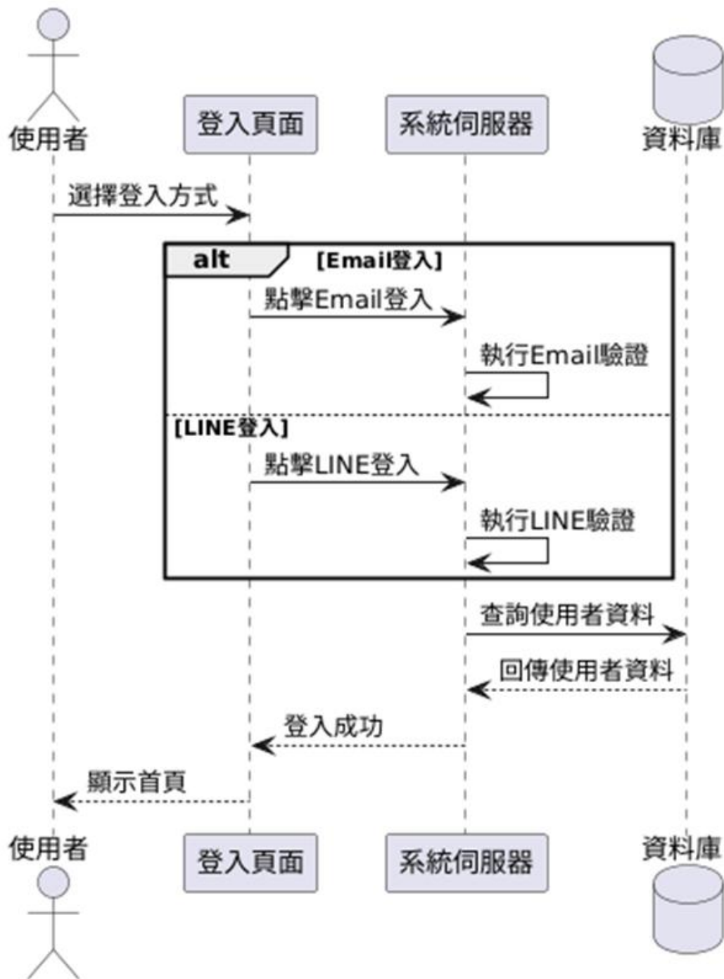
圖 6-1-1 登入循序圖
