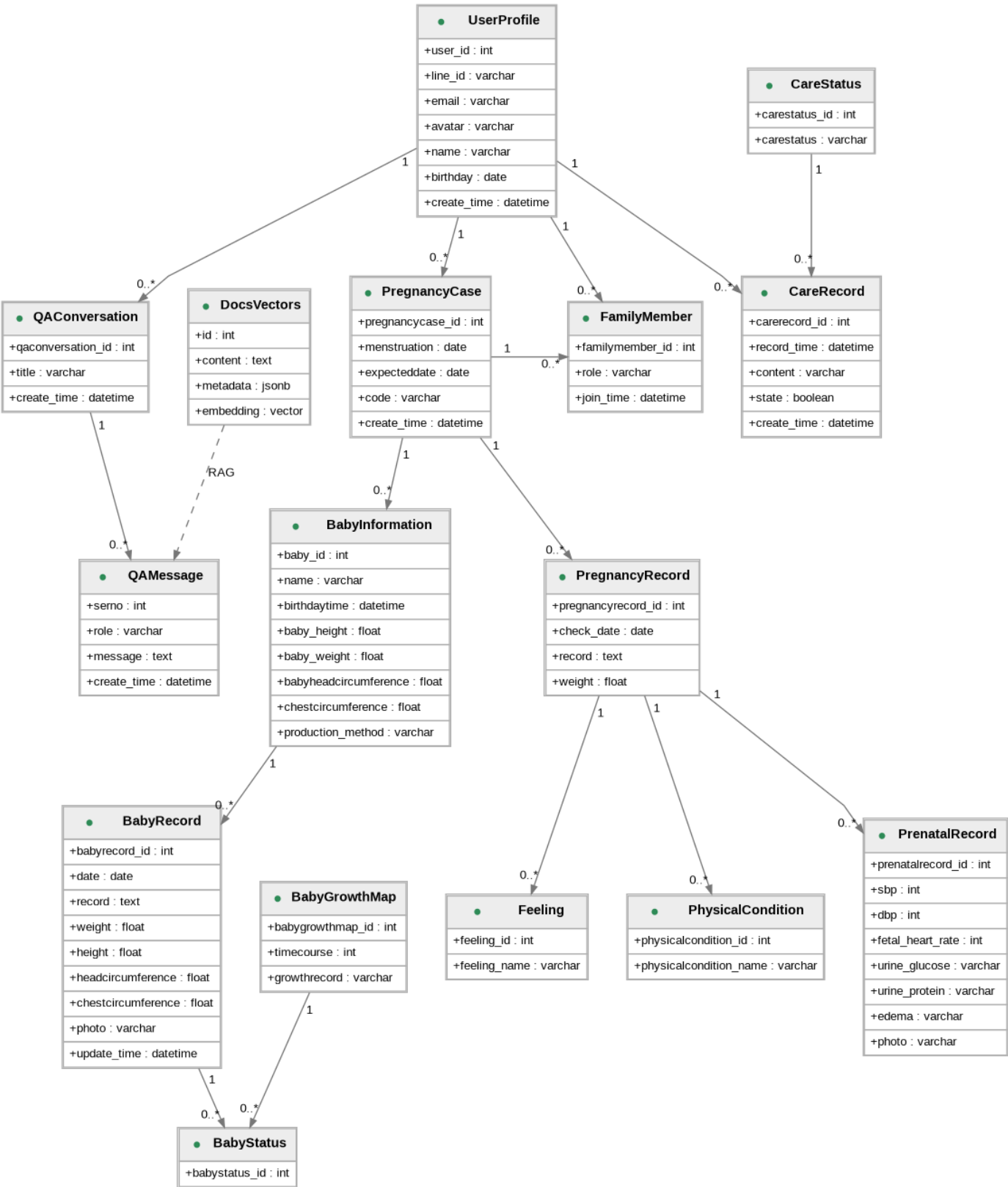
圖 5-4-1 分析類別圖
