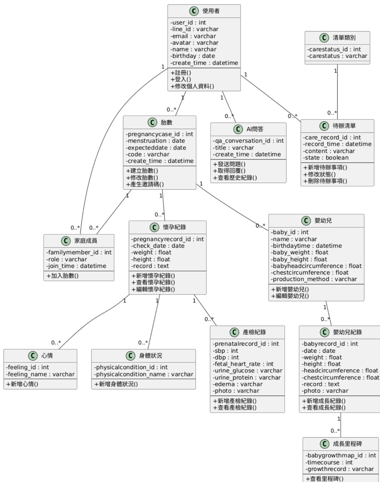
圖 6-2-1 設計類別圖
