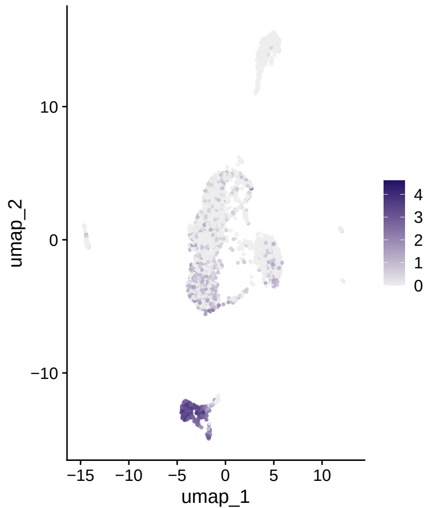
NKG7
