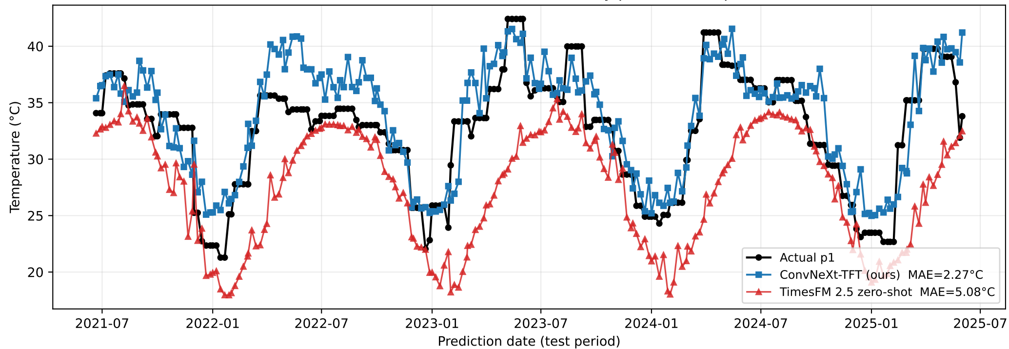
Center (Tel Aviv) — month-ahead hottest day p1: actual vs predicted
