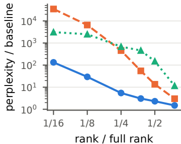
OLMo-2-0425-1B
