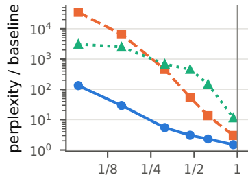
OLMo-2-0425-1B
