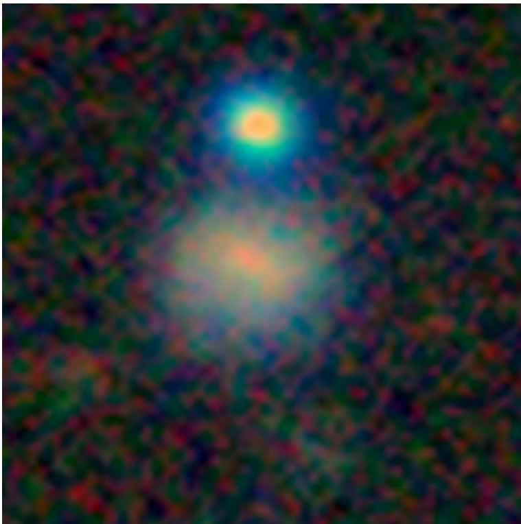
BGS
