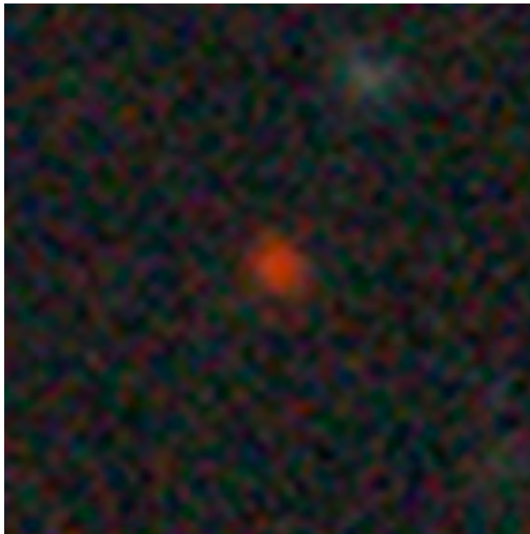
LRG
