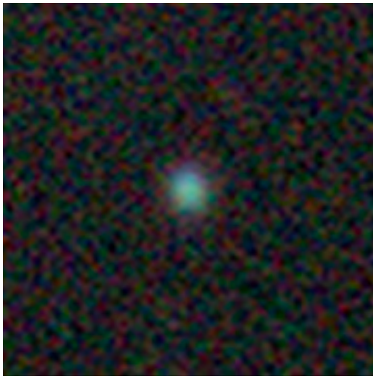
QSO
