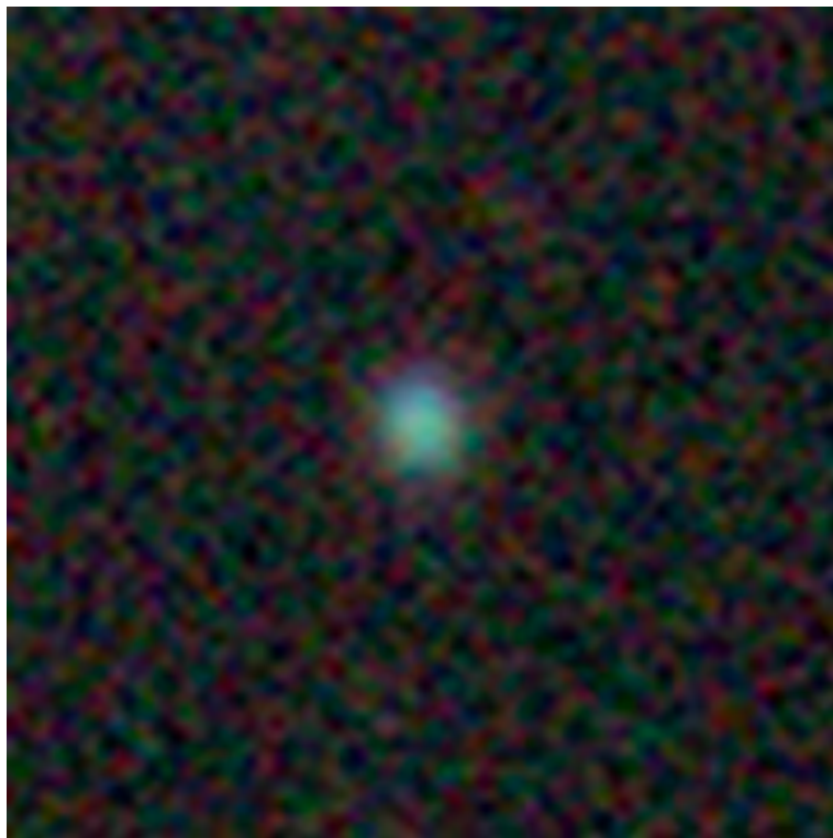
QSO
