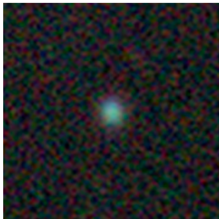
QSO
