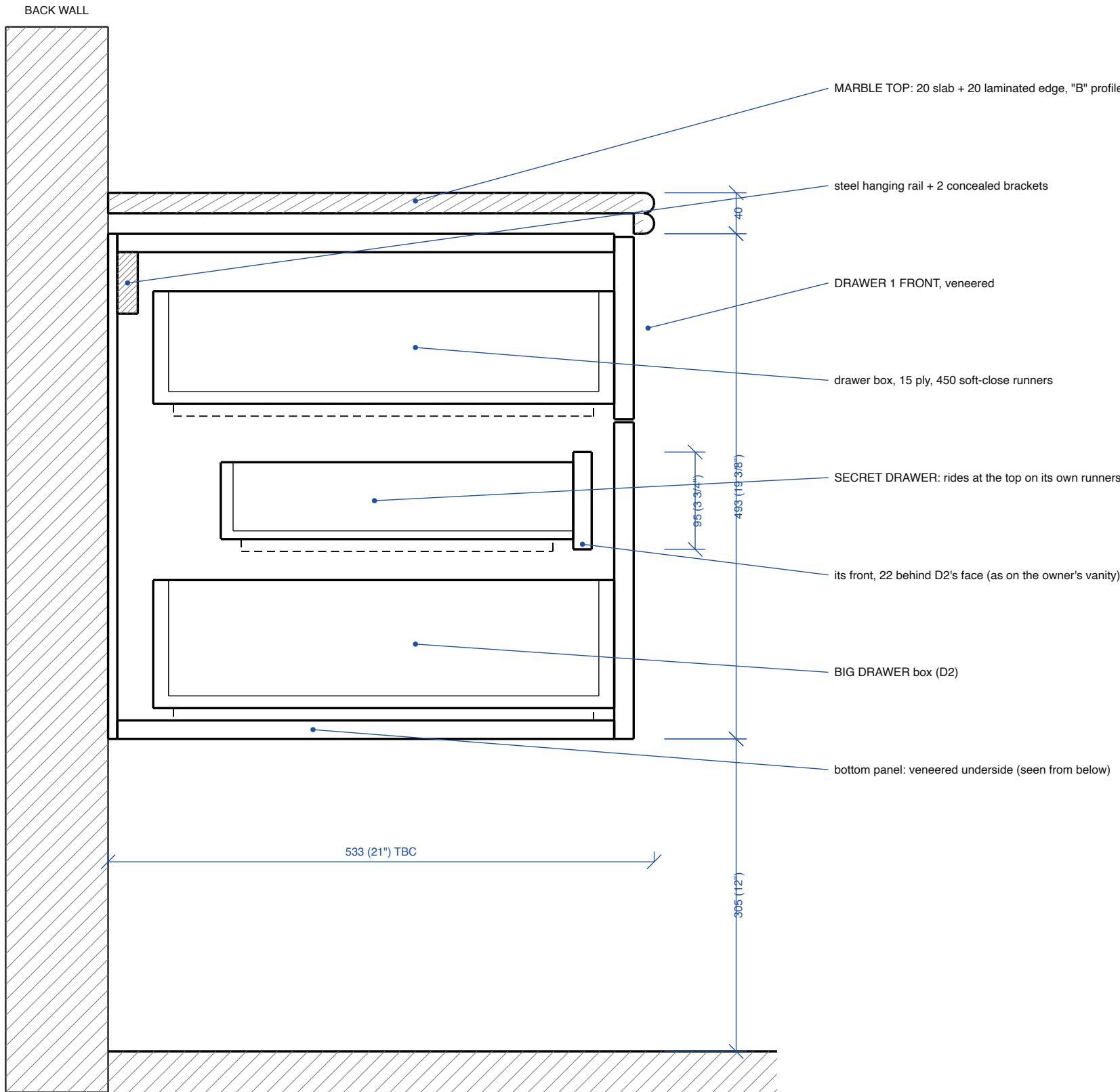
SECTION A-A
